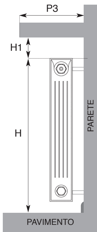
VISTA LATERALE CON EVENTUALE OSTACOLO SUPERIORE
